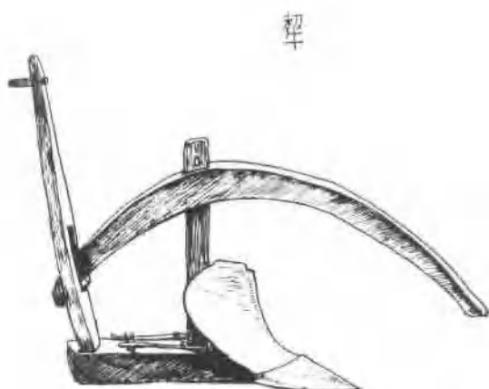
“溪家土角”犁，犁口中长度为3.5寸(市尺)可 入土四寸，只适用于粗放的耕作方法。
