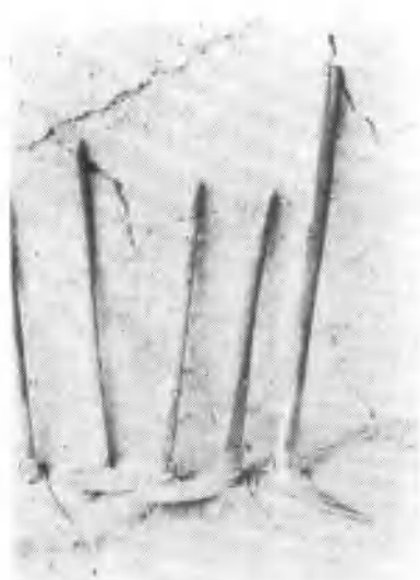
凉山一般使用的尖锄和截锄 (雷波县)
