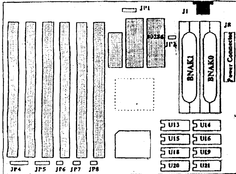
图 1—3 286 主机板结构图
