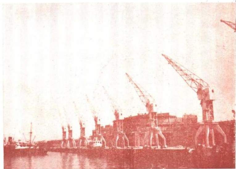
圖十三 叙利亞西部拉塔基亞新港的建設工地，新港的建設始于1952年11月，預定1957年年底完成，据叙利亞官方公布的材料，新港建成后，将是东地中海的最大港口之一
