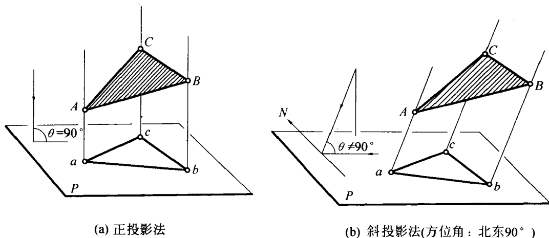
图 1-3 平行投影法
