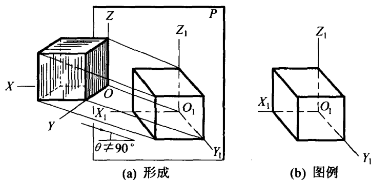
图 1-11 斜轴测图
