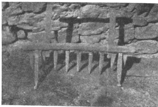
木 耙 (紅河)
