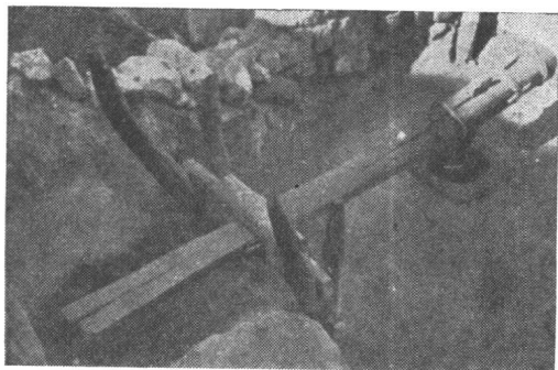
木 碓 (紅河)
