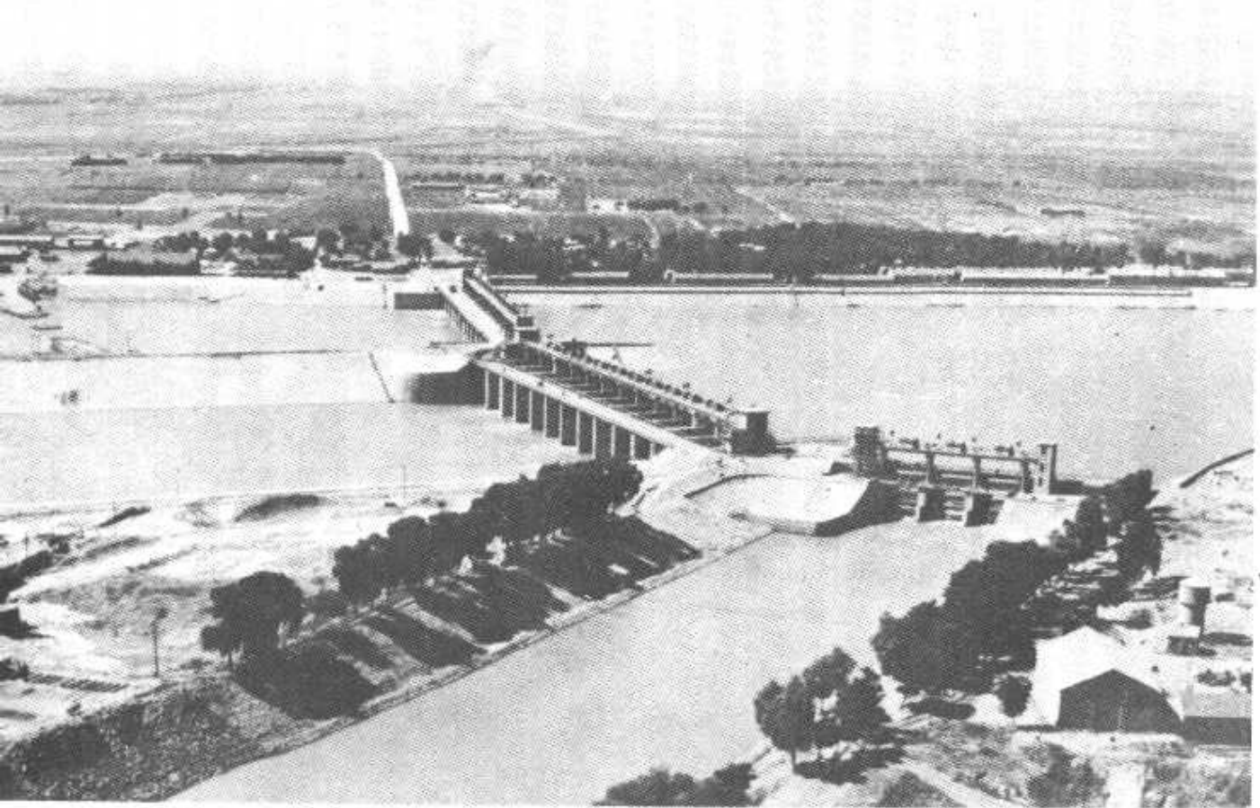
雄伟壮观的子牙新河“穿运”枢纽工程(上图)和四女寺枢纽工程(下图)。
