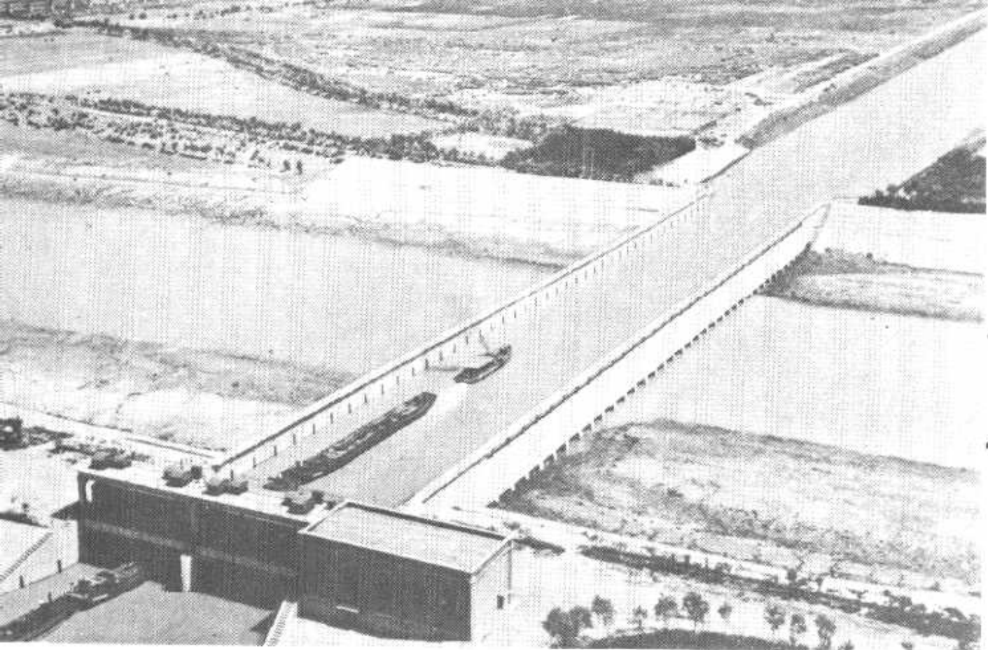
雄伟壮观的子牙新河“穿运”枢纽工程(上图)和四女寺枢纽工程(下图)。
