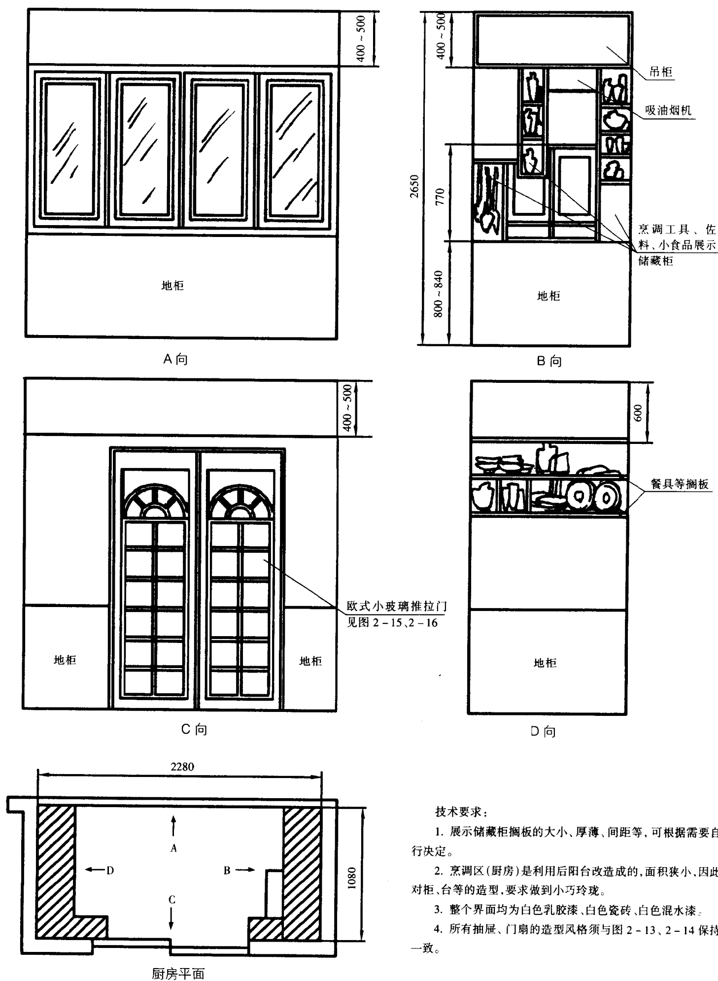
图 2-11 厨房四周界面功能规划
