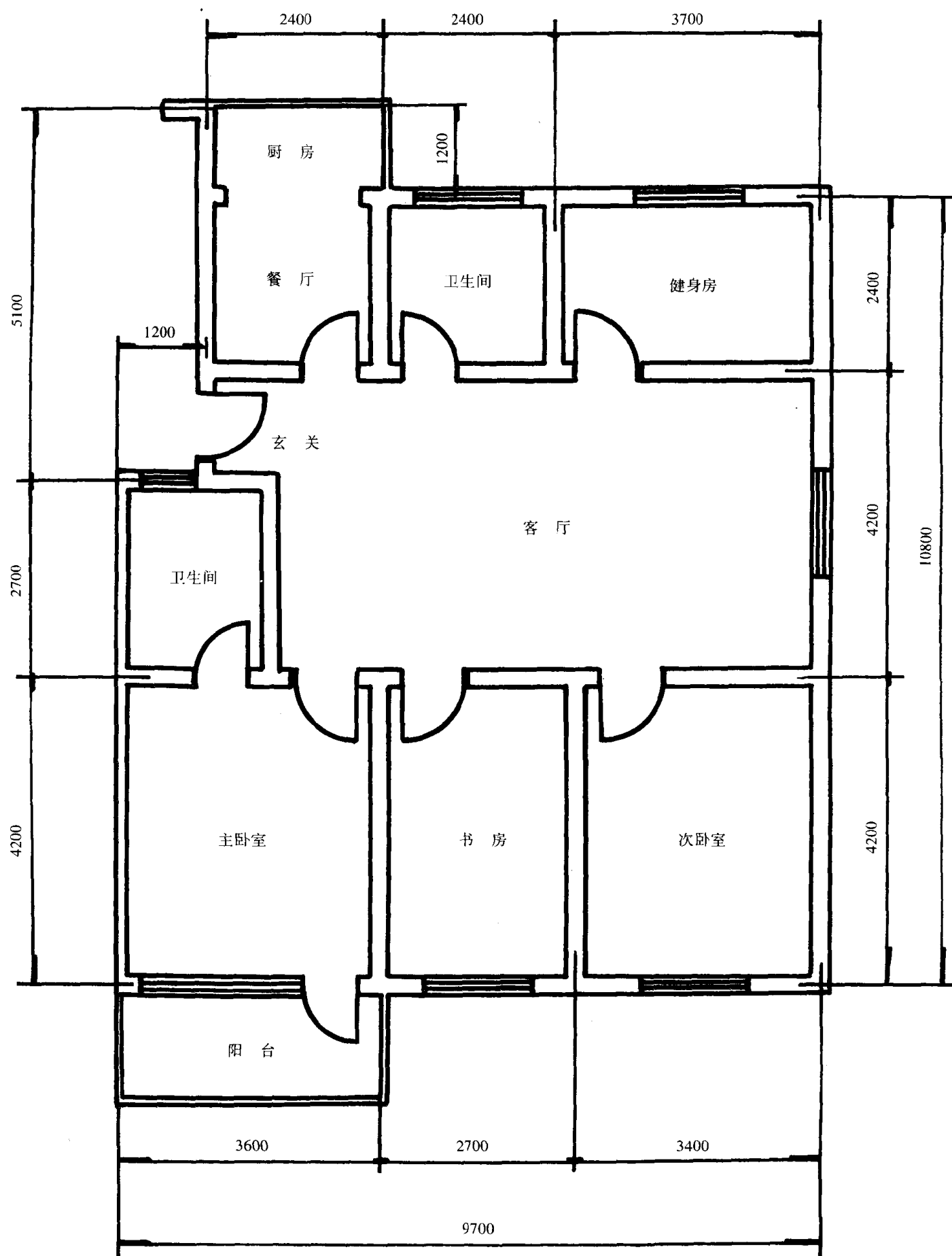
图 2-9 居室平面图(建筑面积 114 m 2 )
