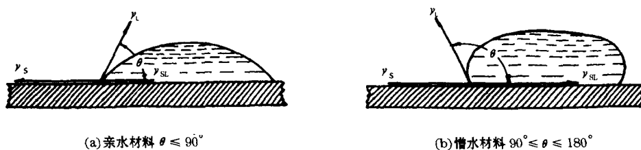
图 1-1 材料的润湿角
