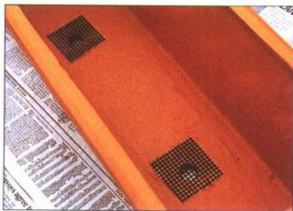
1 在塑料花盆的底部排水孔上放上防止害虫进入的防虫网。
