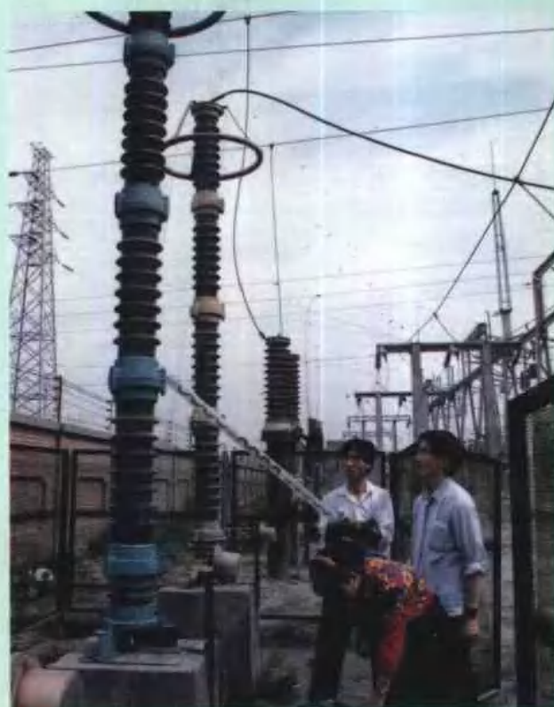
自制 FZ 避雷器带电测试仪
