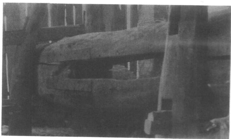
木油榨
