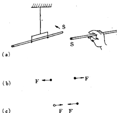
图 1—3 点磁极的相互作用
