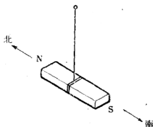
图 1—2 悬挂起来的条形磁铁
