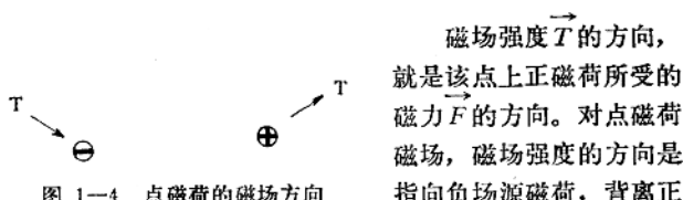
图 1—4 点磁荷的磁场方向
