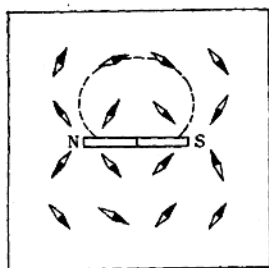
图 1—5 磁铁周围的磁场特征
