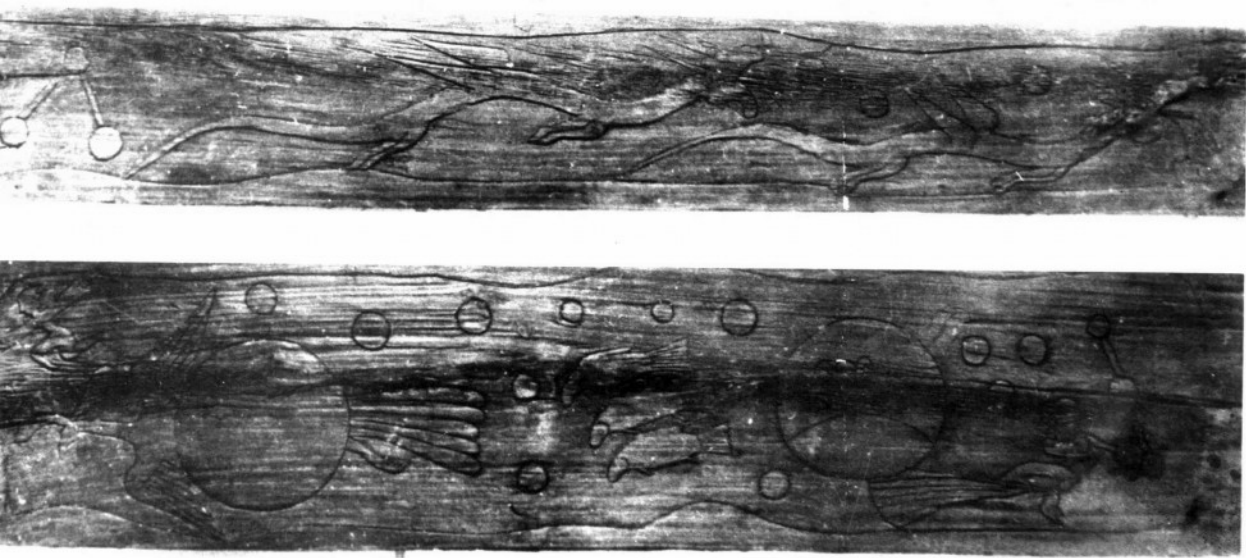
彗星运行图
