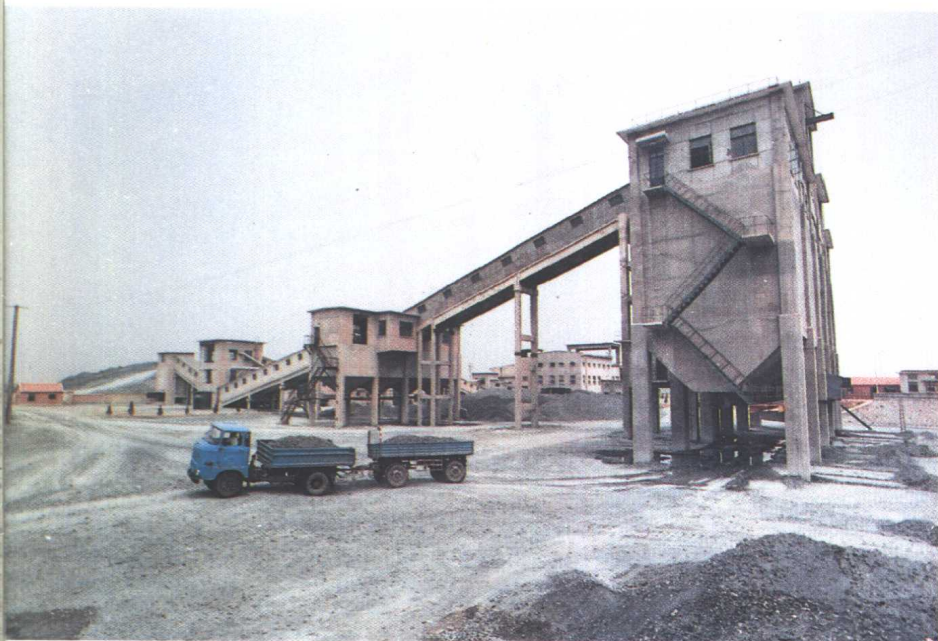
东海蛇纹石矿
