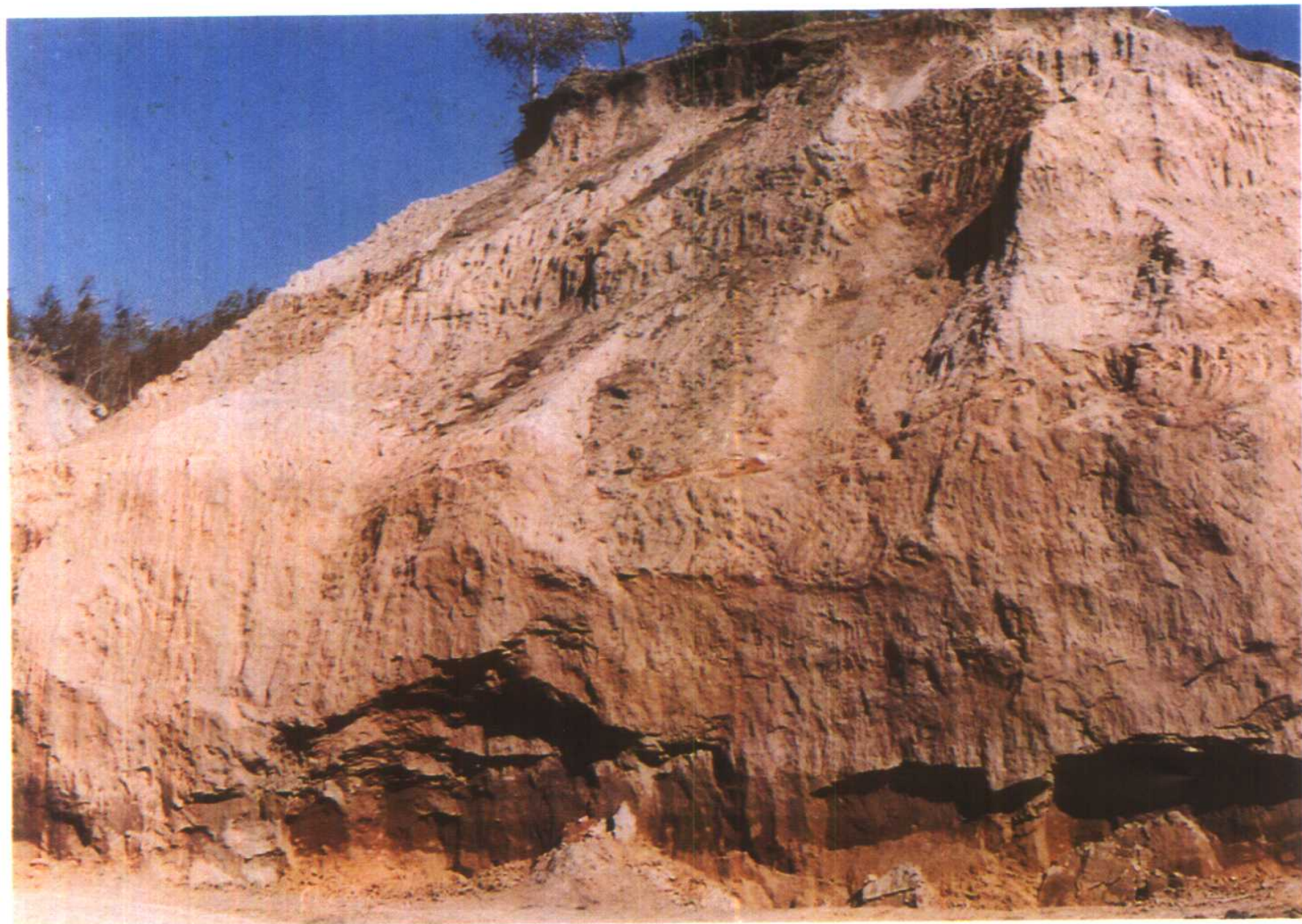
图版 4 荒山剖面（上部为哈尔滨组，中部为上荒山组，下部为下荒山组）
