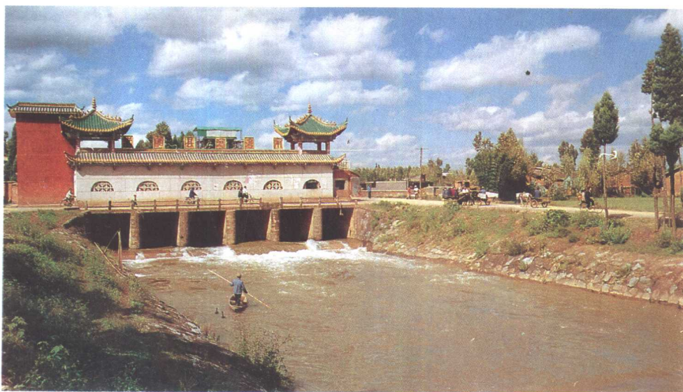
▶ 果马河河湾桥闸
