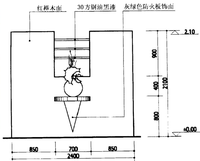
玄关 A 立面展开图
