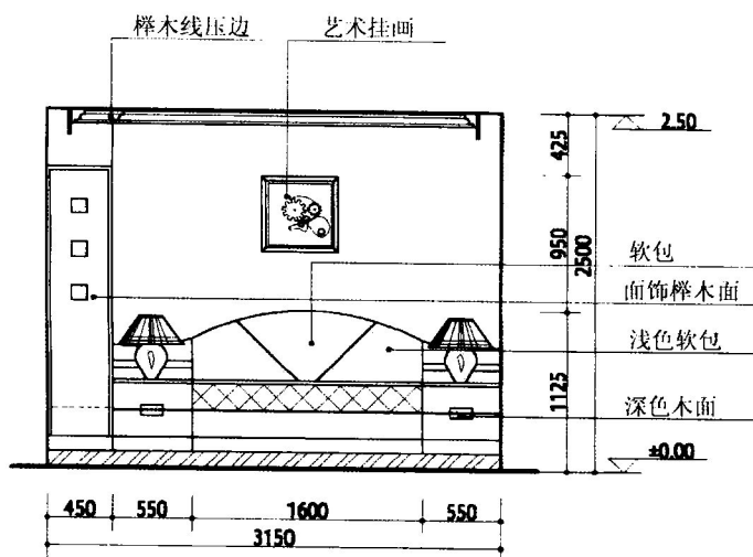
卧室 E 立面图
