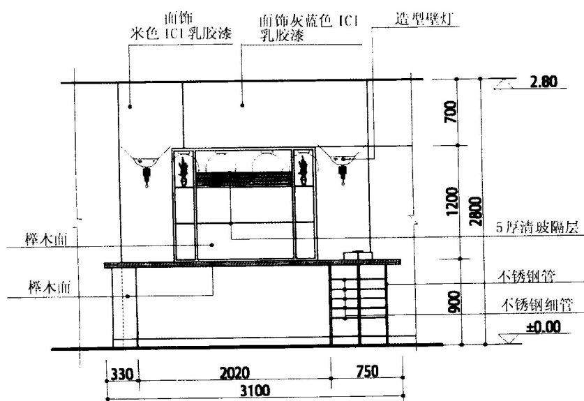
吧台 C 立面图
