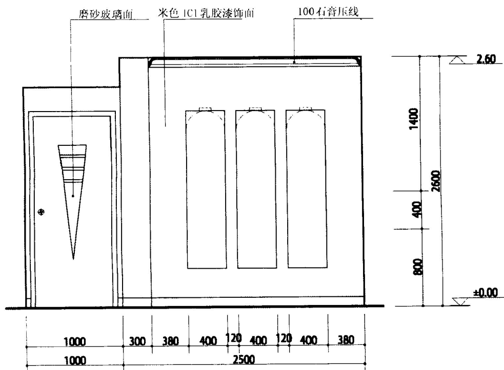
客厅B立面展开图
