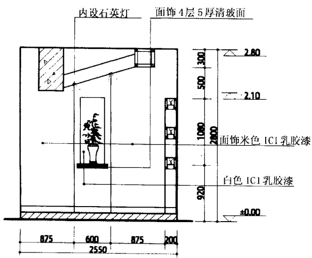
和室 D 立面图
