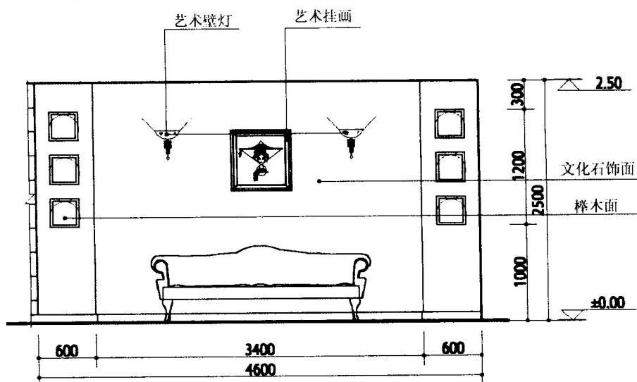
客厅 A 立面图
