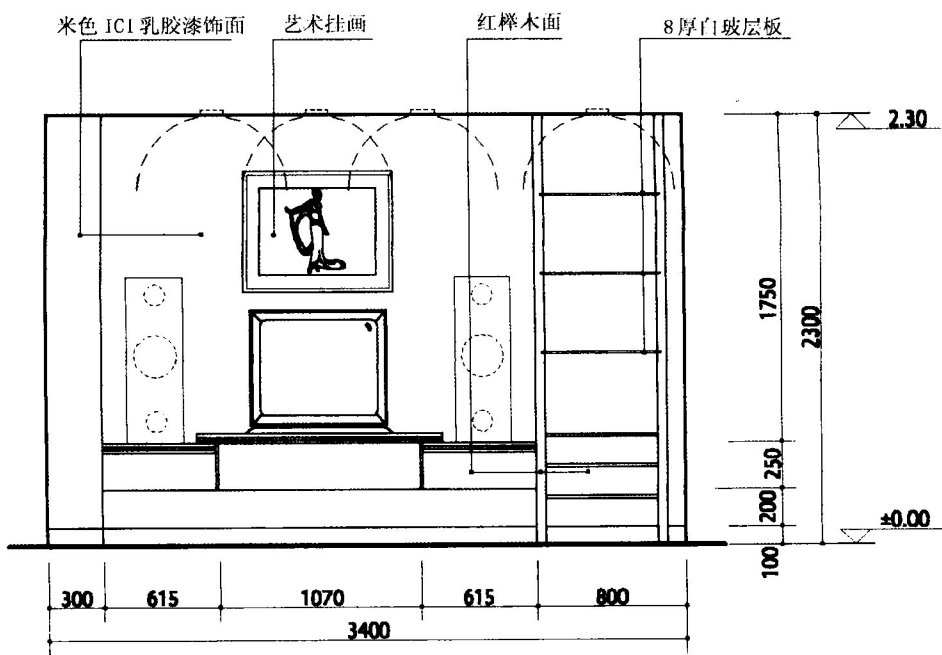
客厅 C 立面图
