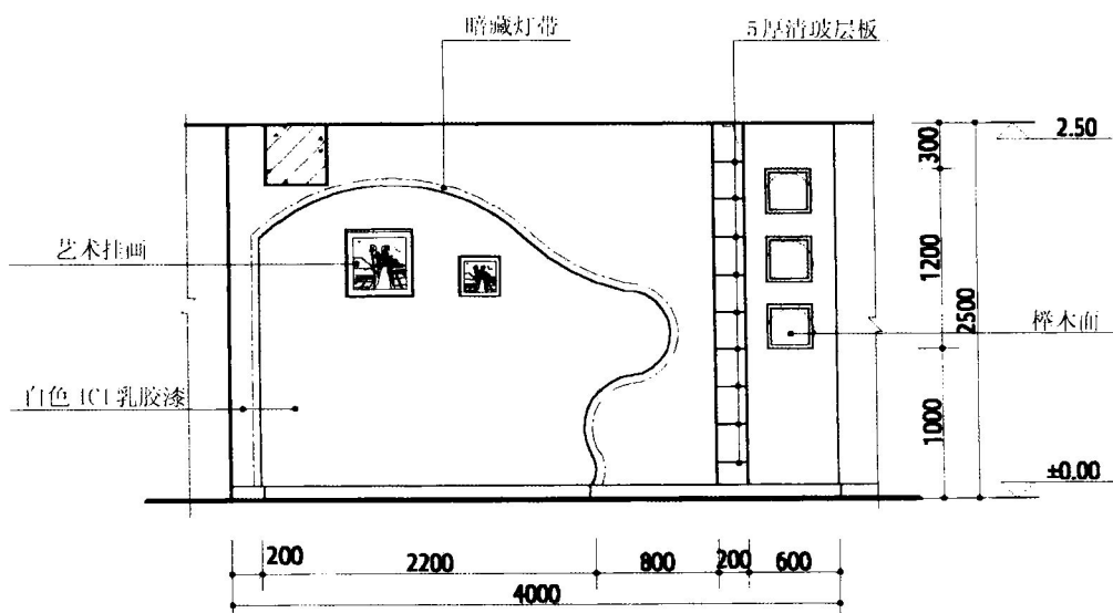
客厅 B 立面图
