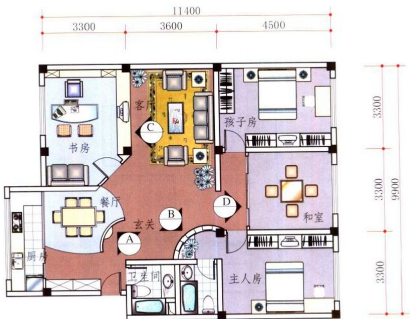
平面布置图 scale 1:150
