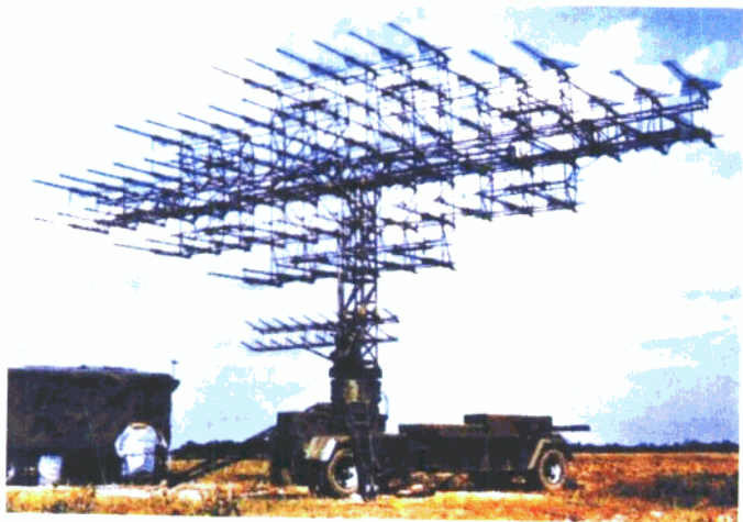
中国远程警戒雷达
