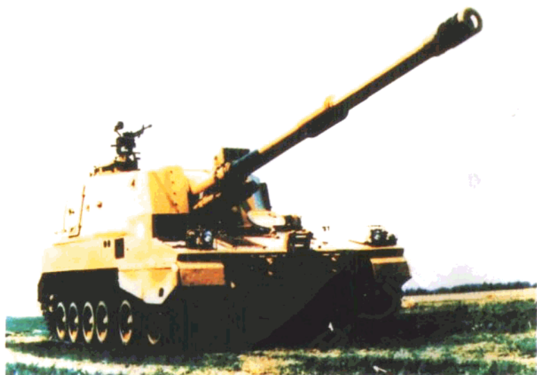
中国 155 自行榴弹炮
