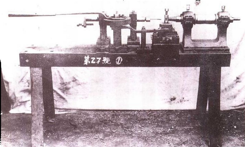
上图为抗战时期子弹厂用道轨钢自制的切口机。
