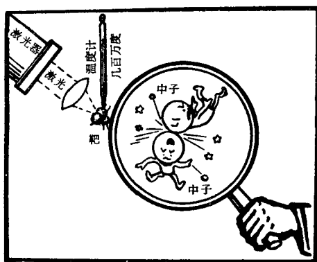
图4 激光引发热核反应
