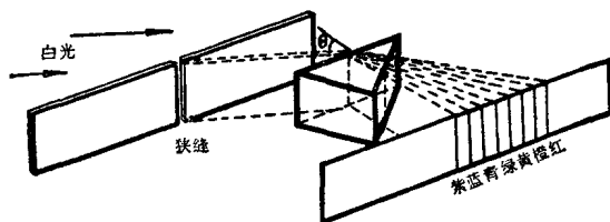
图7 三棱镜分光
