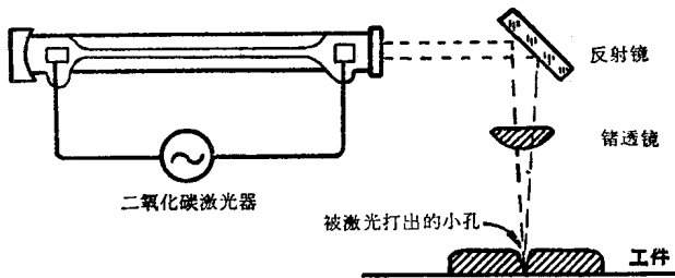
图 2 激光打孔
