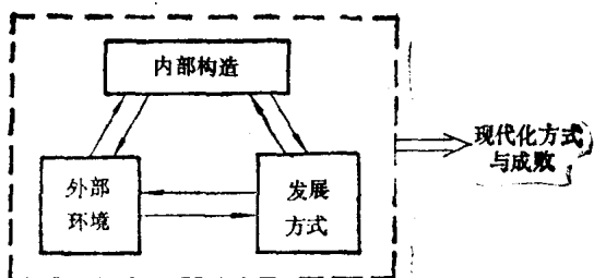
图1 “三体问题”图示
