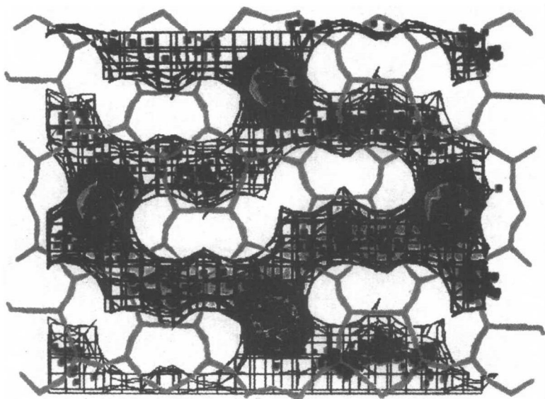
铯在低铝沸石中运动的分子模拟 (■是铯的质心)
