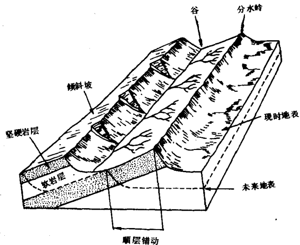
图1-1 示明分水岭和河谷在形态、成因和发展方面关系的图块
