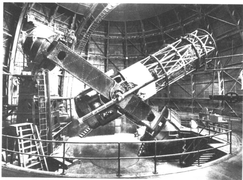
100英寸(2.54米)胡克望远镜,它的镜筒与水平面成 40^\circ 角。哈勃使用的弯木椅可以穿过栏杆看到。
