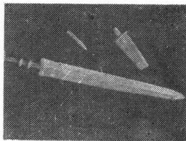
铜剑和箭镞
