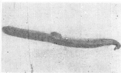
铜带钩
