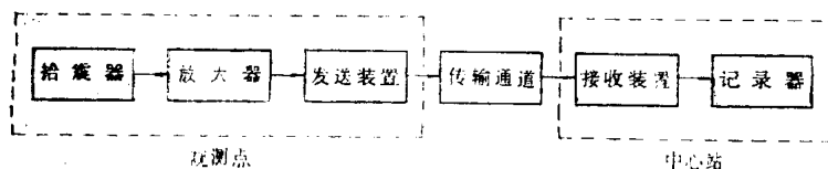
图A.1 地震遥测系统方框图
