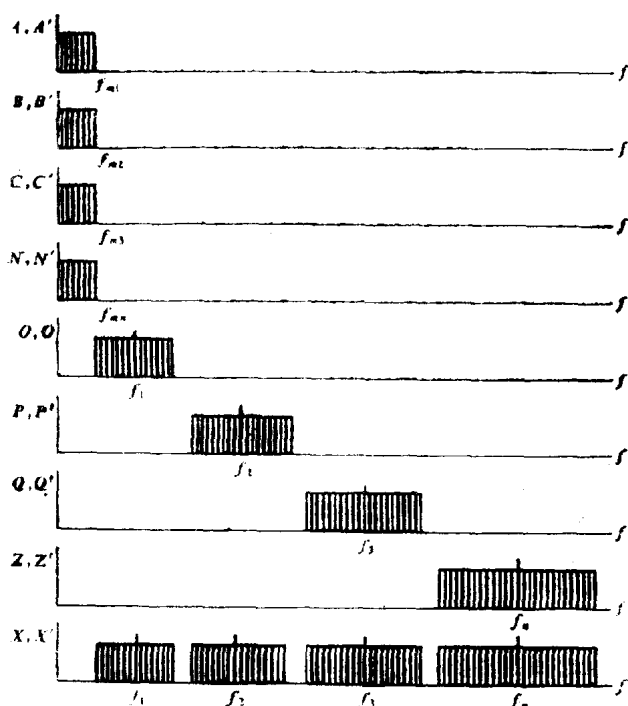
图A.3 图A.2中各点的信号频谱图
