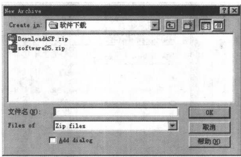
图 1-13 新建对话框
