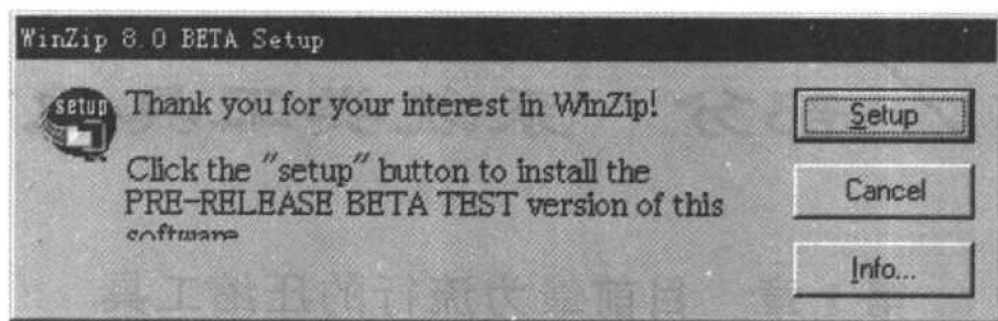
图 1-1 Setup 对话框
