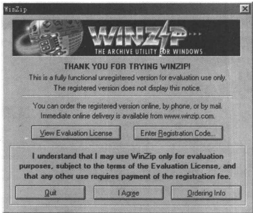
图 1-5 注册对话框
