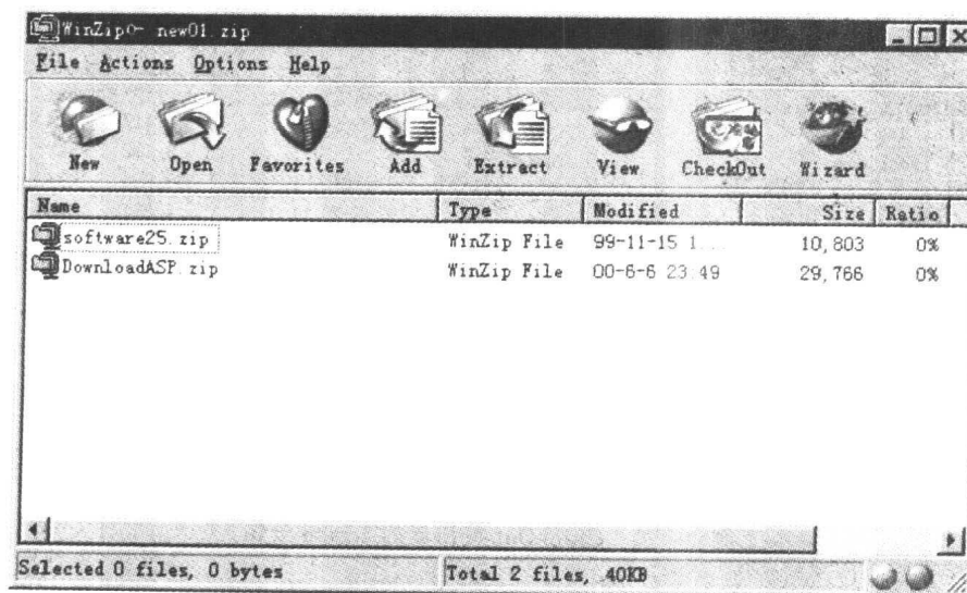
图 1-15 主窗口界面
