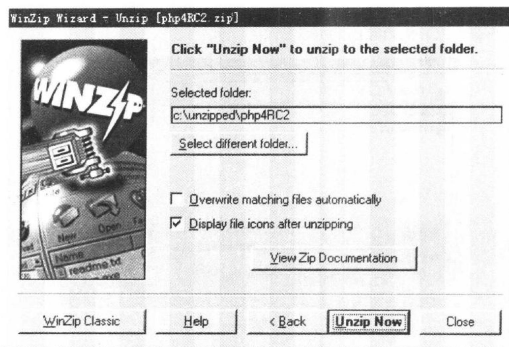
图 1-11 解压缩界面
