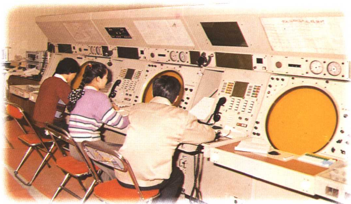
80 年代安装的航管雷达系统
