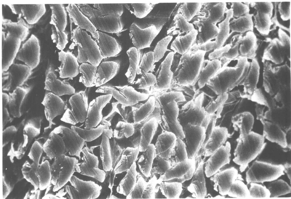
图片二 丝纤维横截面切片投影
