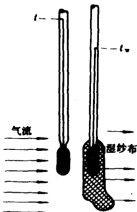
图 1-1 干湿球温度计
