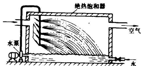
图 1-2 绝热饱和器
