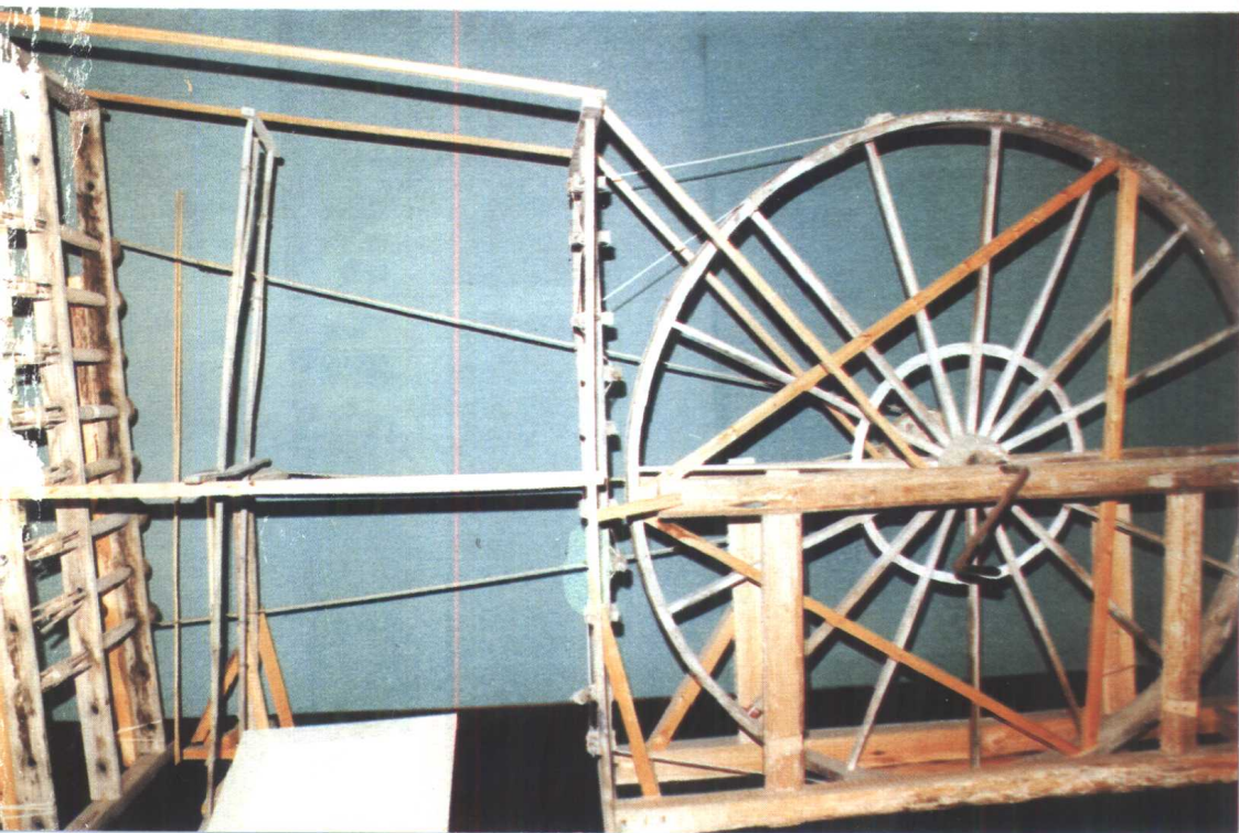
大纺车
