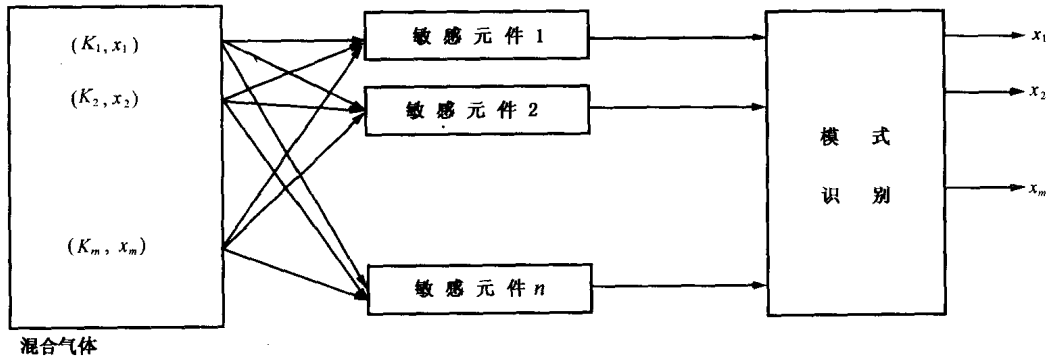
图 1-3 人工嗅觉系统结构图
