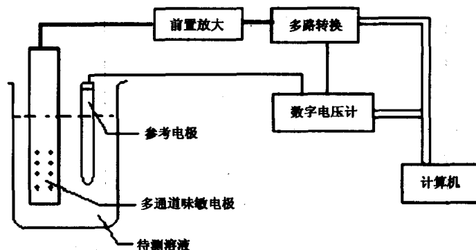
图 1-4 一种多通道人工味觉实验装置
