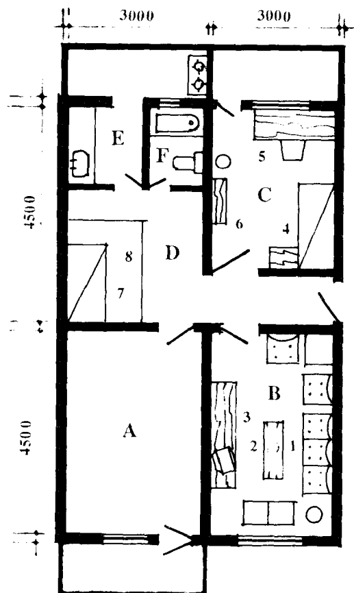
平面布置图
