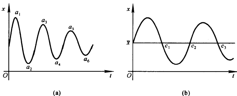
图 1.1.1-7 光点振动位移-时间曲线
