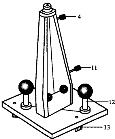
图 1.1.1-4 卡文迪许型扭秤的外形
