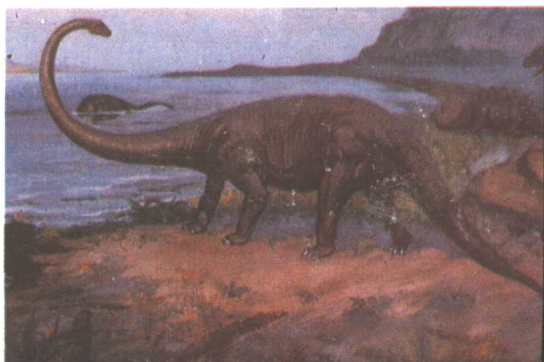
四川恐龙 ⇨
