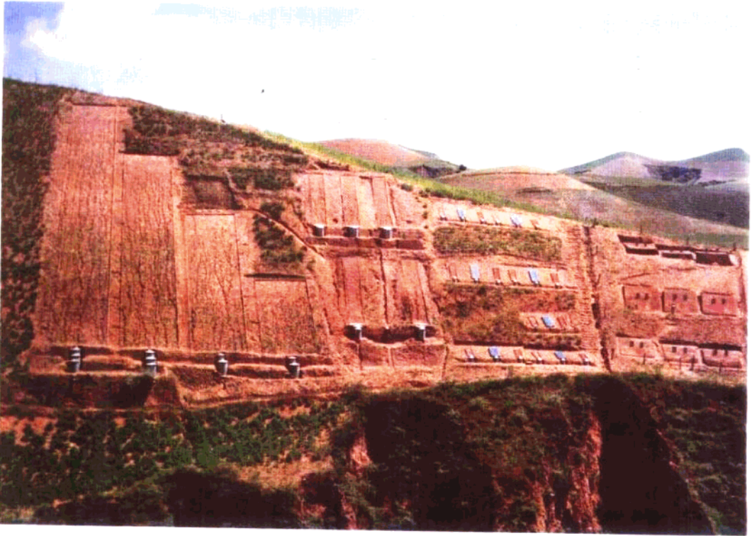
安塞水土保持综合试验站山地侵蚀试验场
