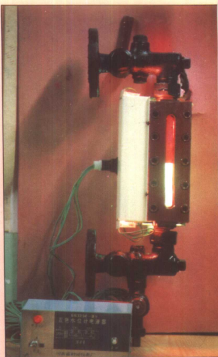
双色水位计
