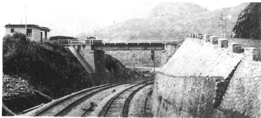
荔波应昂煤矿修建的公路铁路交叉桥
