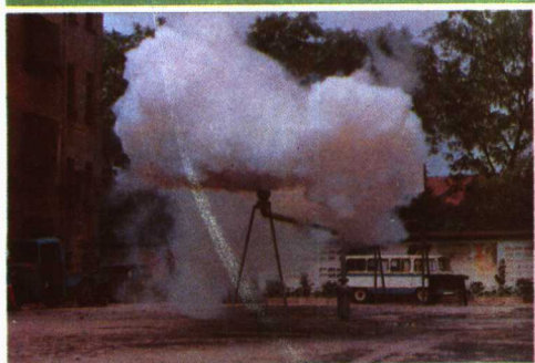
罐外式烟雾自动灭火试验
