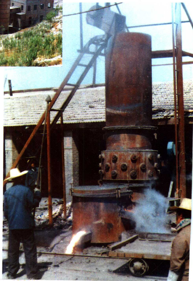
山城村铸造厂化铁炉
