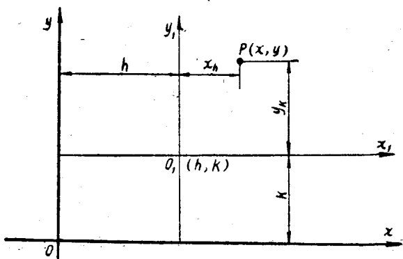
图21-4 坐标的移动变换
