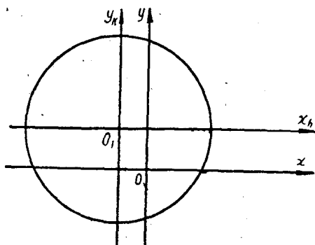
图21-5 圆的坐标平移举例
