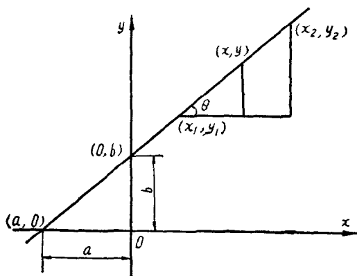
图21—1 二元一次方程的图形是直线
