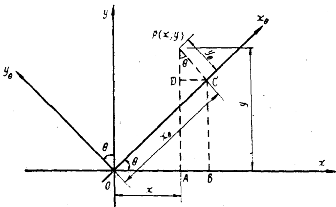
图21-6 坐标转动变换
