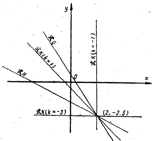
图21-2 二元一次方程组的求解
