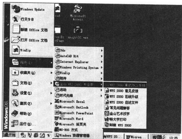
图 1-1 安装 WPS 2000
