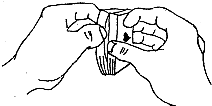
图 4 交错洗牌
