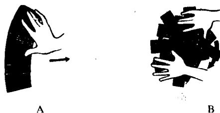
图 1 圆式洗牌法
