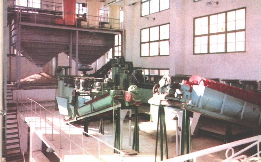
型砂厂精选车间
