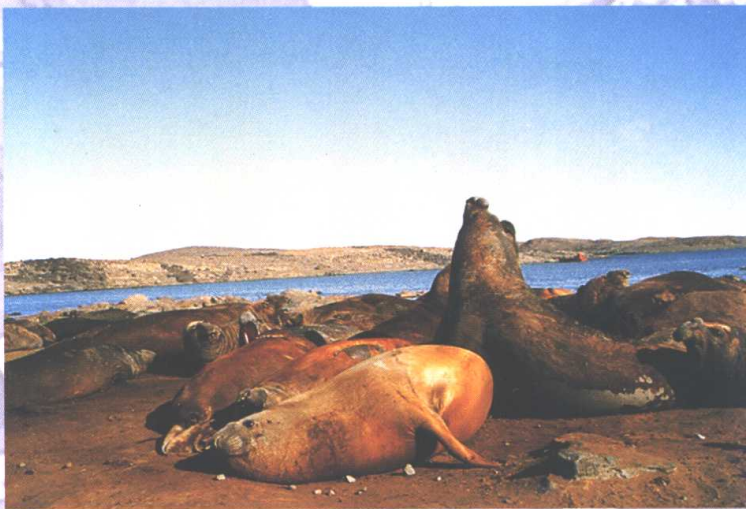
南极象海豹 ▶
