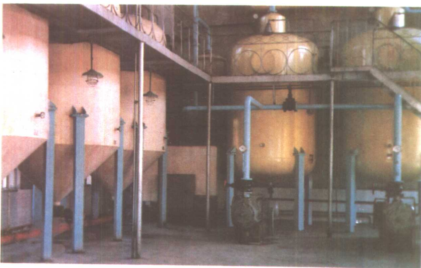
80年代制油设备（水化罐、真空脱臭罐）
