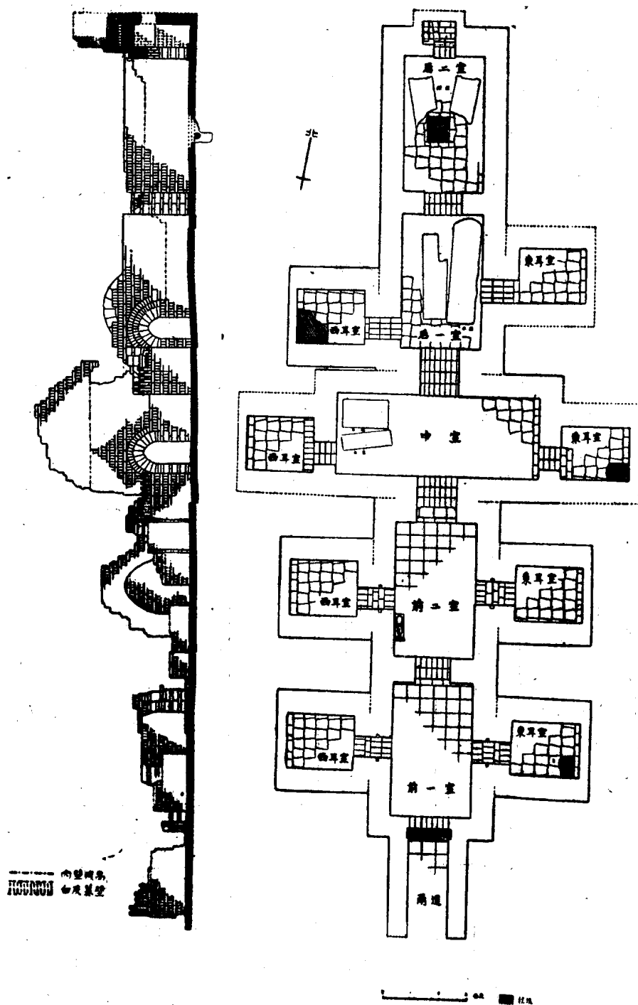
插图二 望都二号汉墓墓室平面、剖面图
