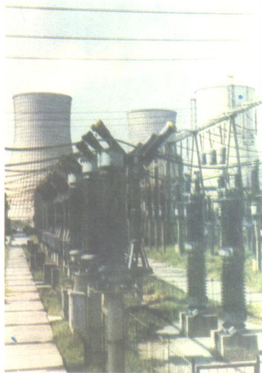
火电厂超高压变电站
