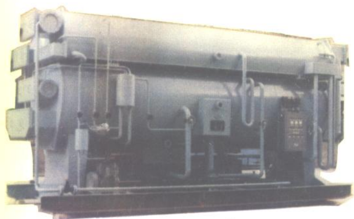
通用机械厂生产的150型蒸汽两效溴化锂吸收式制冷机
