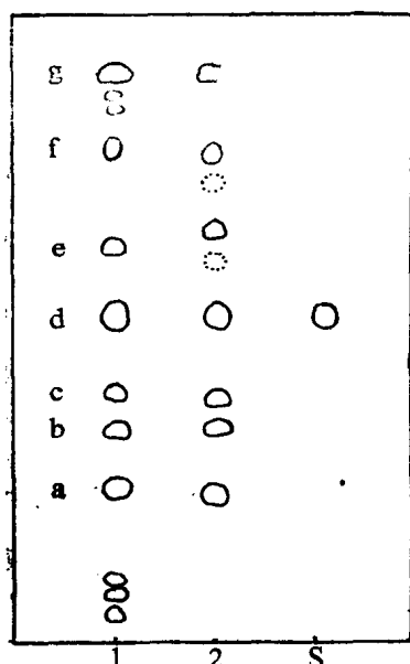
图 4-1 八珍丸(甘草)薄层色谱图
