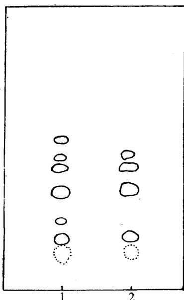
图 3-1 十香返生丸(苏合香) 薄层色谱图
