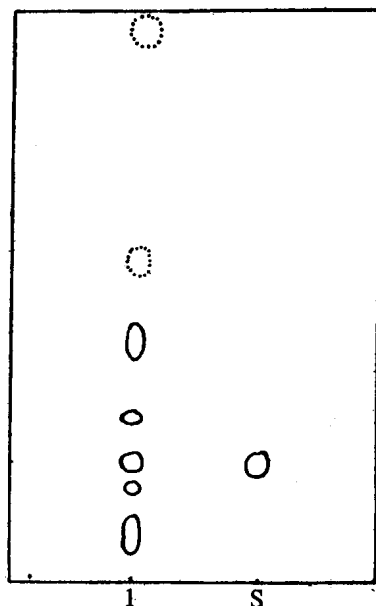
图 3-2 十香返生丸(牛黄)薄层 色谱图
