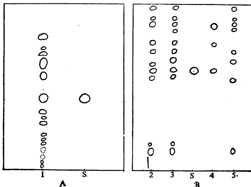
图 2-1 十全大补丸(白芍)薄层色谱图
