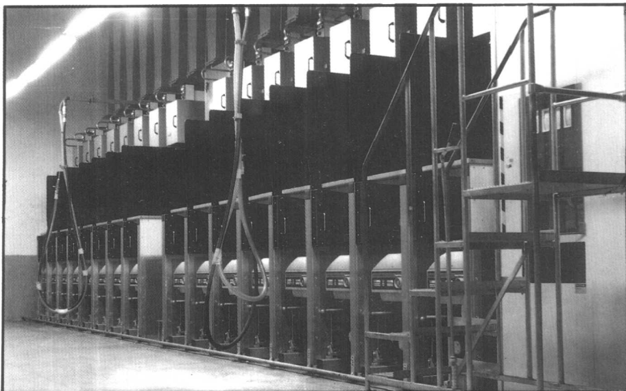
凯里涤纶厂从 德国引进的仿真丝 生产线
